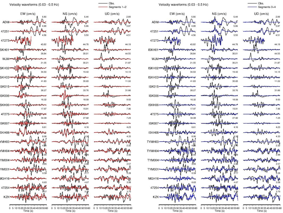
図 4: 地震①(左)と地震②(右)の波形への奇与
