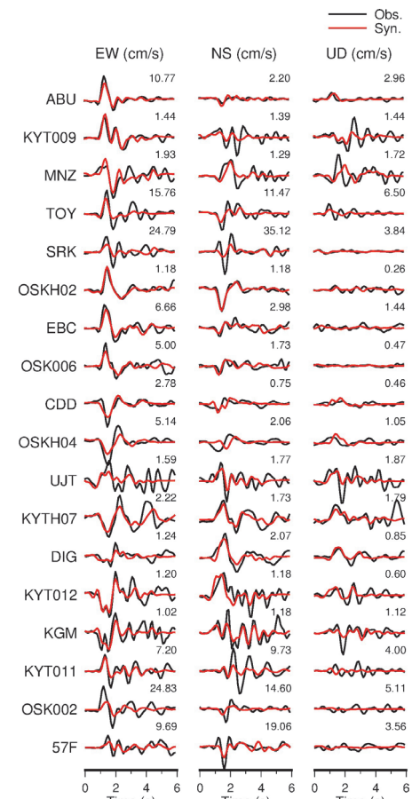
図 4 速度波形(0.1~1.5Hz)の比較 (黒: 観測、赤: 合成)
