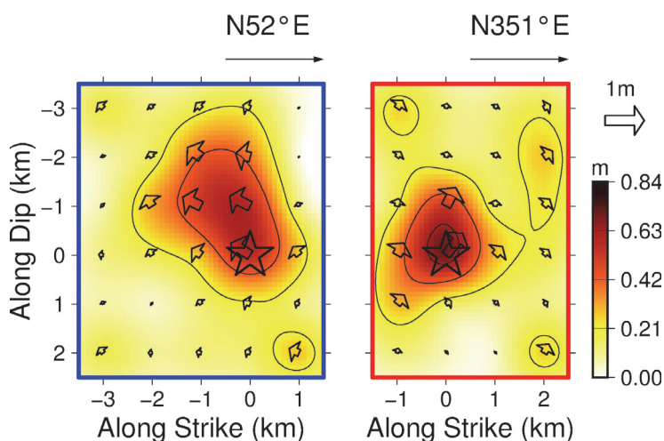
図 3 最終すべり分布 (☆: 共通の破壊開始点)
