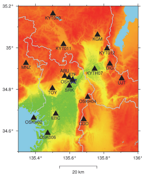
図 1 観測点(▲)及び震央(★)
