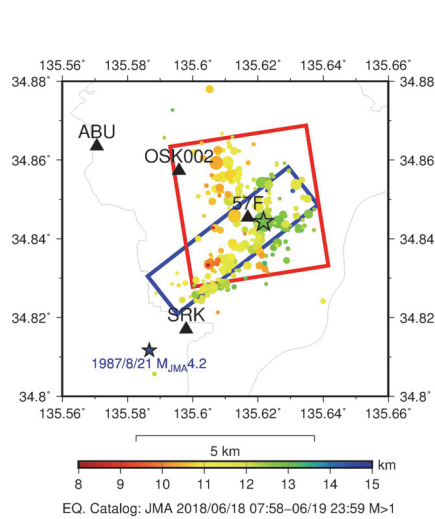
図 2 断層面の地表投影及び余震分布
