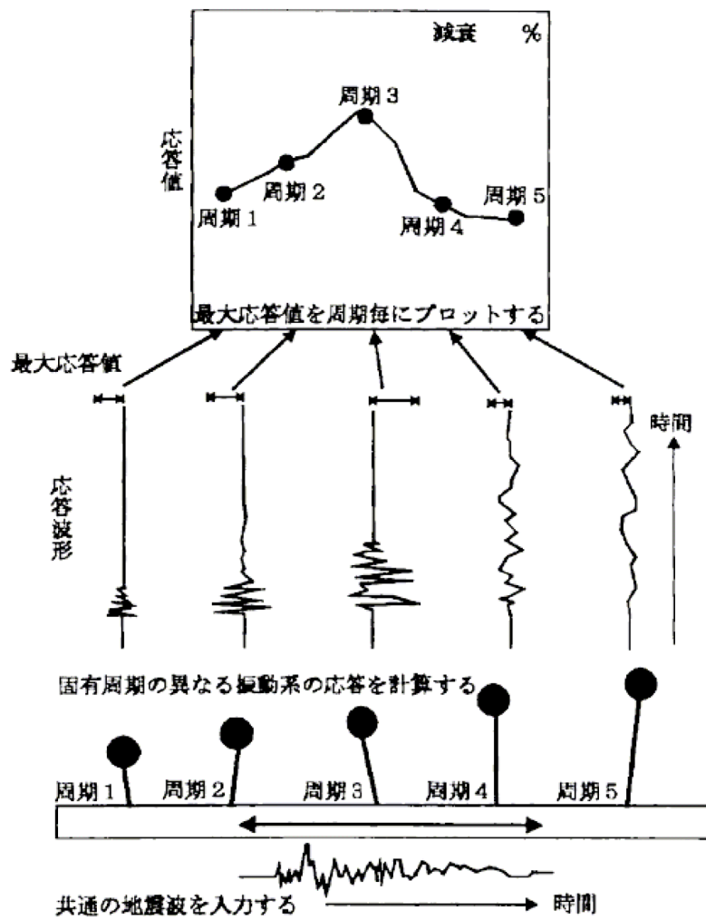
図 2-2.2 応答スペクトルの概念
