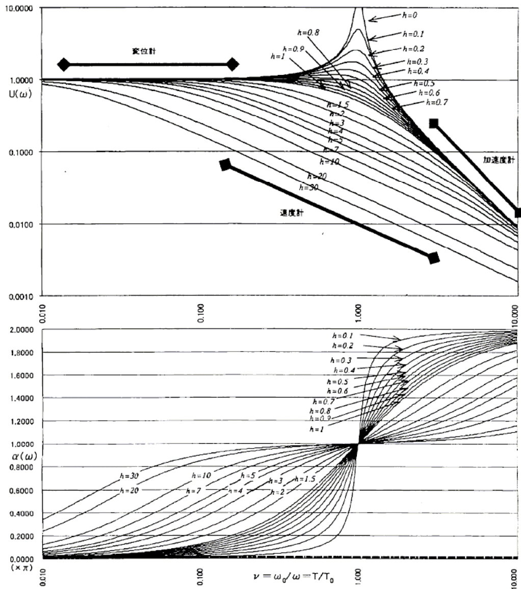
図 2.1.2 地震計の振幅と位相の周波数特性
